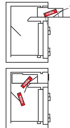
Modèle Zephir Dépôt 802. Avec tiroir sur le côté gauche.
